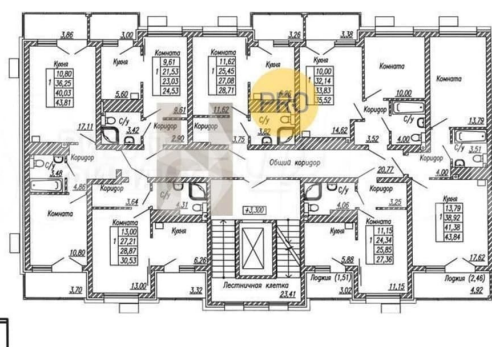
КОРПУС 9 Секция 1 План 2-7 этажей
