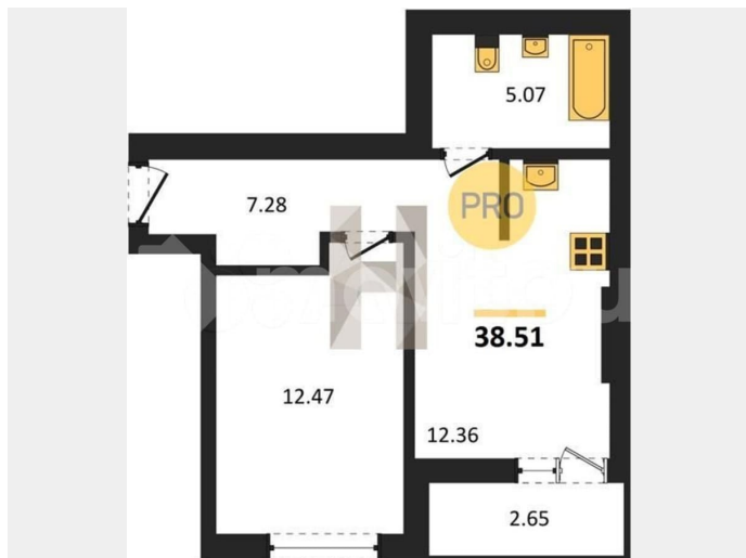
КОРПУС 3 Секция 1 План 1-4 этажей
