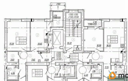
КОРПУС 7 Секция 2 План 2-5 этажей
