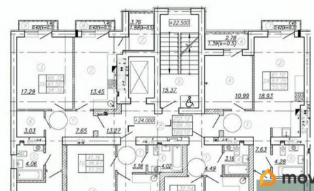
КОРПУС 7 Секция 1 План 9 этажа
