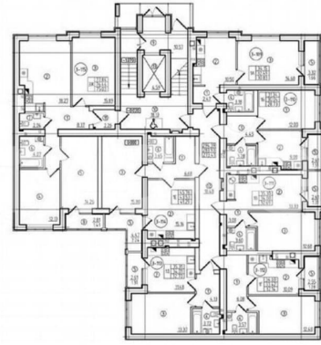
КОРПУС 5 Секция 3 План 1-5 этажей
