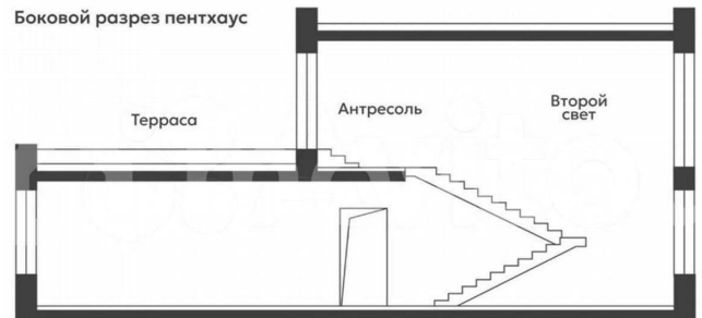
Боковой разрез пентхауса
