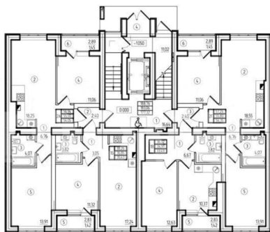
КОРПУС 3 Секция 1 План 1-5 этажей
