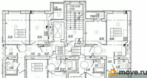
КОРПУС 7 Секция 3 План 6-8 этажей
