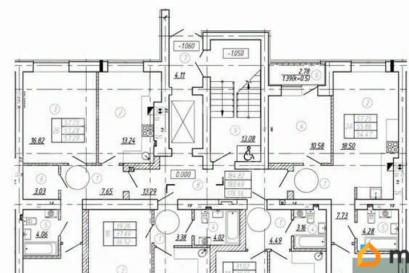
КОРПУС 7 Секция 2 План 1 этажа
