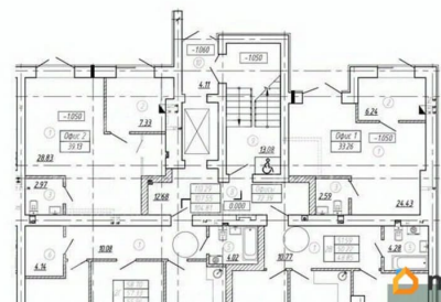
КОРПУС 7 Секция 3 План 1 этажа
