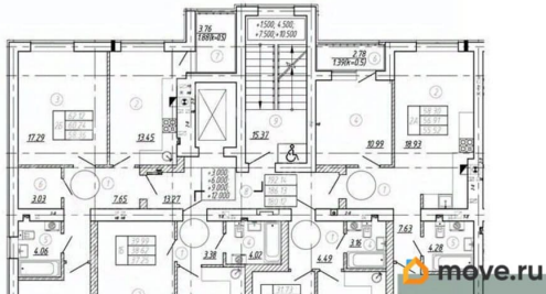
КОРПУС 7 Секция 1 План 2-5 этажей
