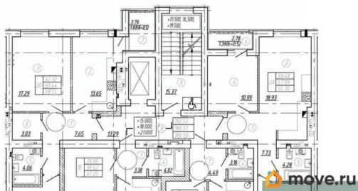
КОРПУС 7 Секция 2 План 6-8 этажей
