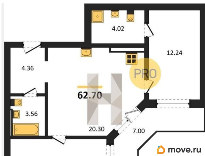
КОРПУС 8 Секция 1 План 1-7 этажей
