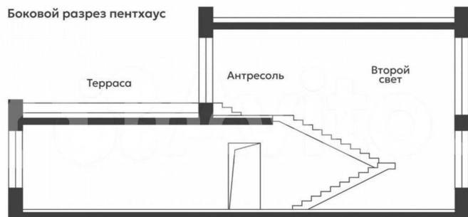
Боковой разрез пентхаус
