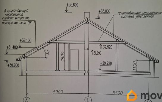
Разрез 1-1
